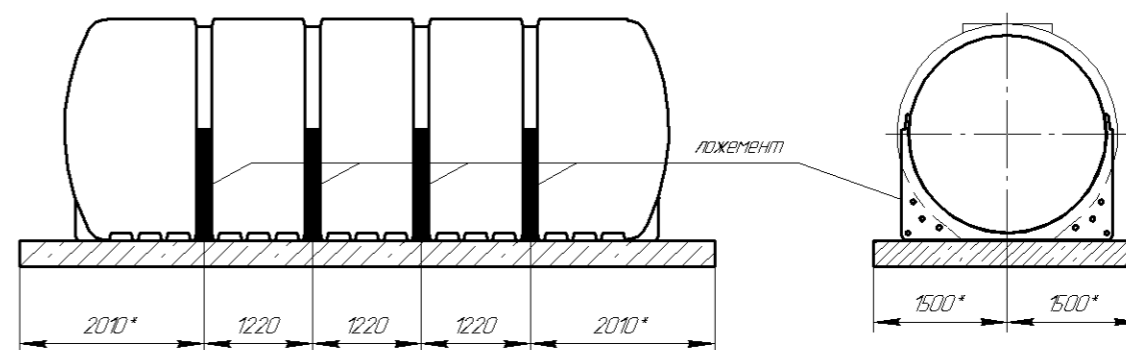
Схема установки ложементов
