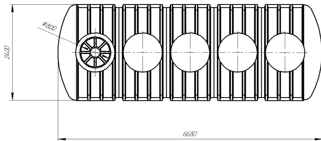
вид А
