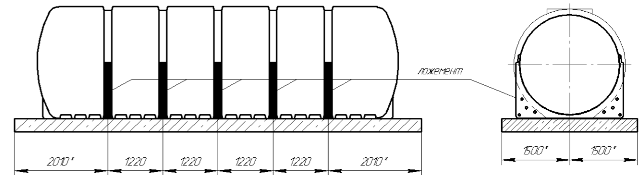
Схема установки ложементов
