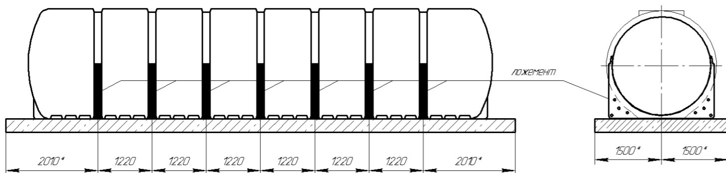
Схема установки ложементов
